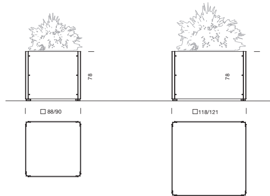
Plaza planter 0,90 m x 0,90 m
