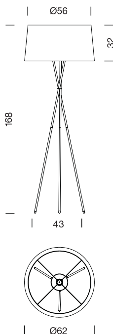
Trípode G5 lámpara de pie
