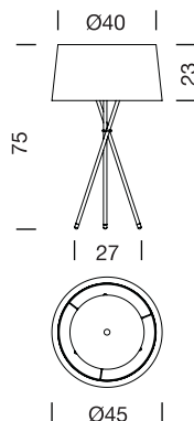
Trípode G6 lámpara de sobremesa
