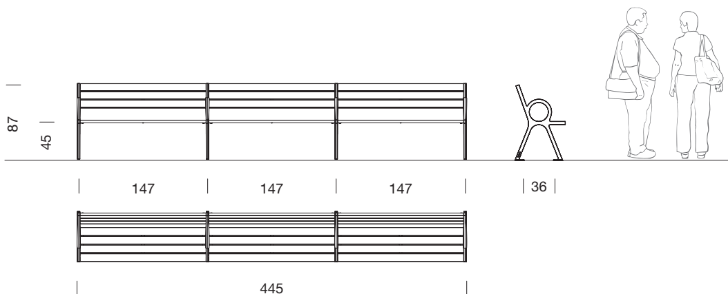
Banco Perisphere de tres tramos con tres respaldos
