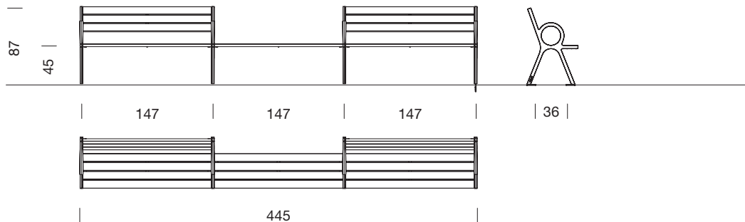
Banco Perisphere de tres tramos con dos respaldos
