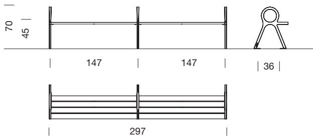
Banco Perisphere de dos tramos sin respaldo
