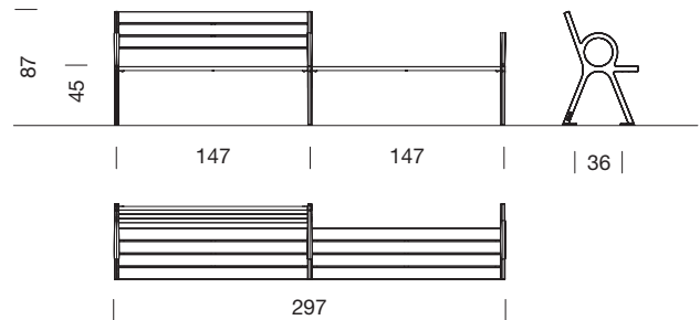
Banco Perisphere de dos tramos con un respaldo inicial
