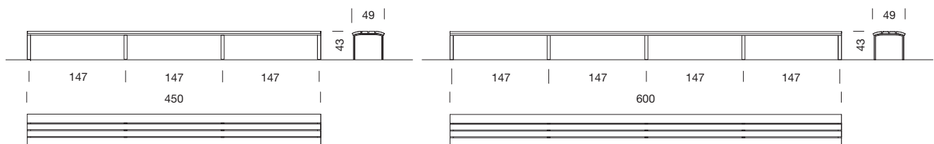
Banqueta NeoRomántico Liviano 100% aluminio de 4,50m
