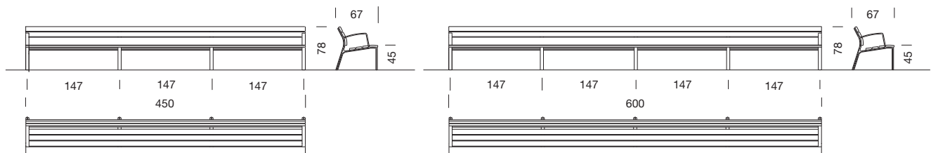
Banco NeoRomántico Liviano 100% aluminio de 4,50m
