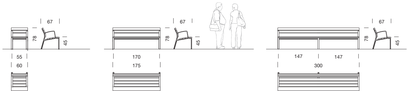
Banco NeoRomántico Liviano 100% aluminio de 0,60m
