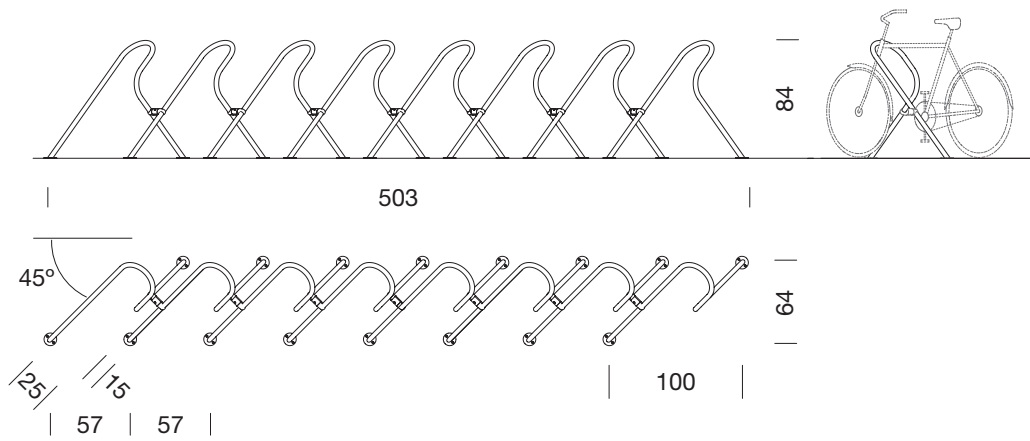
Aparcamiento para bicicletas Montana de 8 soportes
