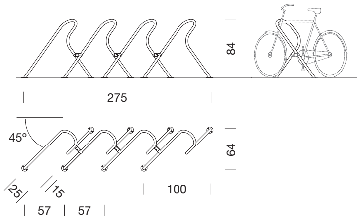
Aparcamiento para bicicletas Montana de 4 soportes
