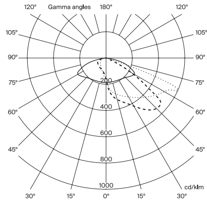
Viaria Distribución TIII LOR 100% ULOR 0%±3%
