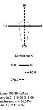
Lámpara HIE-CEm / HSE
