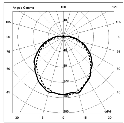
Lámpara HIE-CEm / HSE
