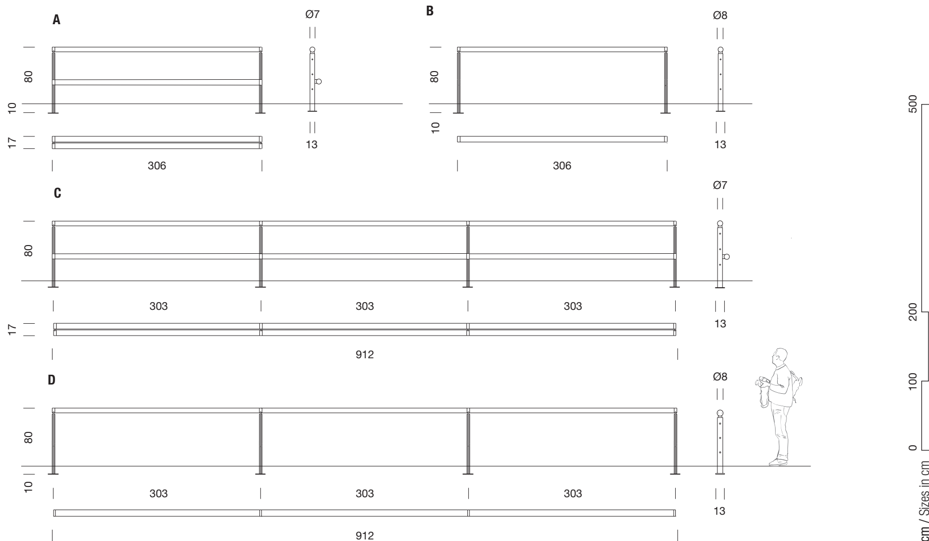
A B C D De un tramo de un tramo con travesaño de tres tramos De tres tramos con travesaño 1 unit 1 unit with crossbeam 3 units 3 units with crossbeam
