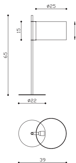
1. TMD lámpara de sobremesa
